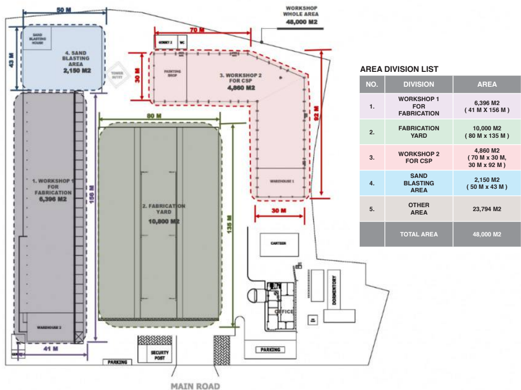
LAYOUT PT. SEPULUH SUMBER ANUGERAH CIKANDE WORKSHOP
